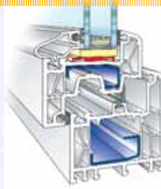
KNIPPING KN0 links mit PROLUX-Flügel rechts mit halbflächen- versetztem Flügel
